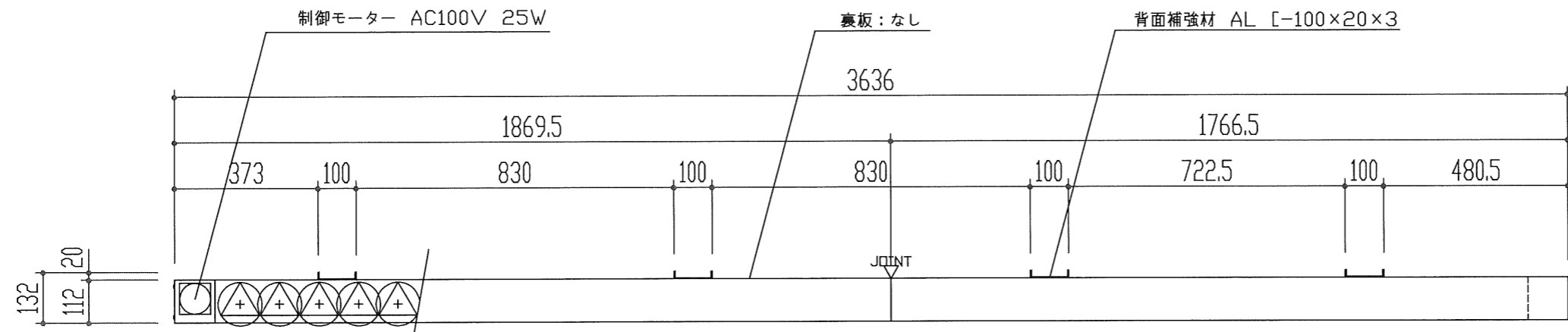
平面図
